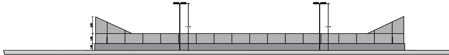
DETALHE - LONGITUDINAL
